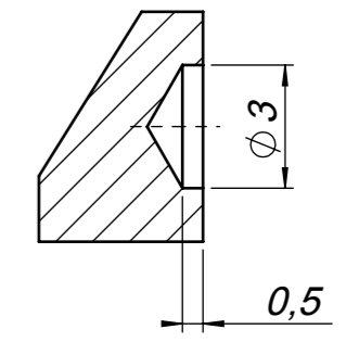
SEZIONE A-A
